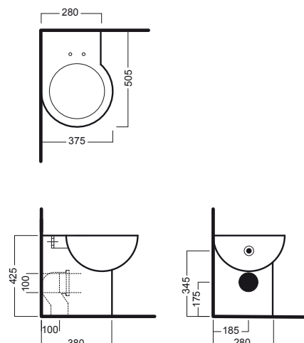
vaso d'angolo destro filo muro back to wall right-hand corner wc
