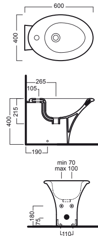
bidet filo muro back to wall bidet
