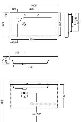
con sifone salvaspazio - with space saver trap_Y1M5
