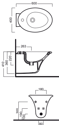
bidet sospeso wall hung bidet
