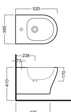
bidet sospeso wall hung bidet
