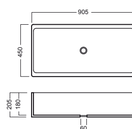
lavabo a canale 90 sink 90
