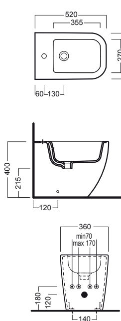
bidet filo muro back to wall bidet
