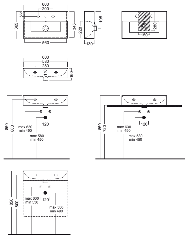
lavabo 60x36,5 washbasin 60x36,5
