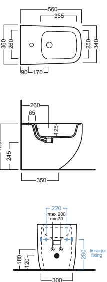
bidet filo muro back to wall bidet
