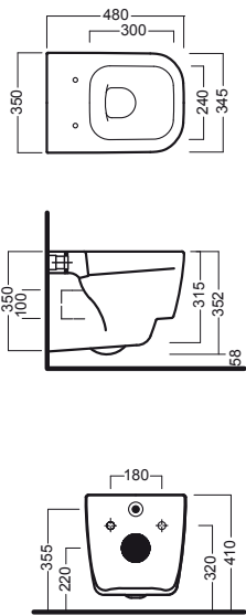
vaso sospeso wall hung wc
