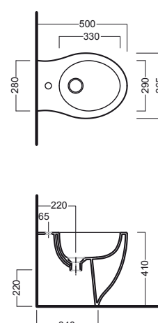
bidet filo muro_50 back to wall bidet_50
