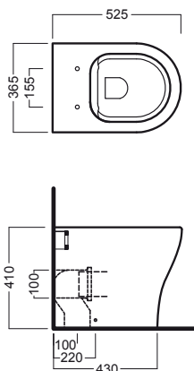
vaso filo muro PURE RIM PURE RIM back to wall wc
