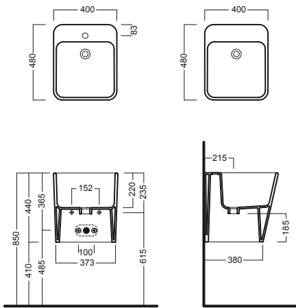
lavabo pilozzo sospeso wall hung sink
