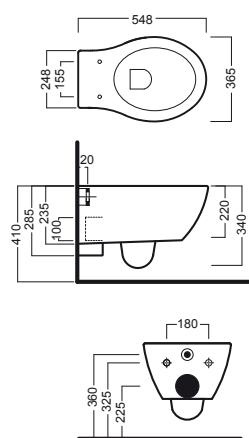
vaso sospeso wall hung wc
