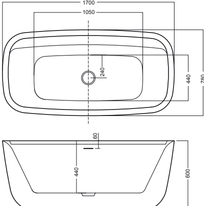
vasca 170x78 BT_03 bathtub 170x78 BT_03
