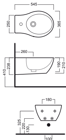
bidet sospeso wall hung bidet
