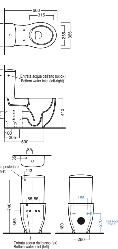
vaso monoblocco PURE RIM PURE RIM coupled wc
