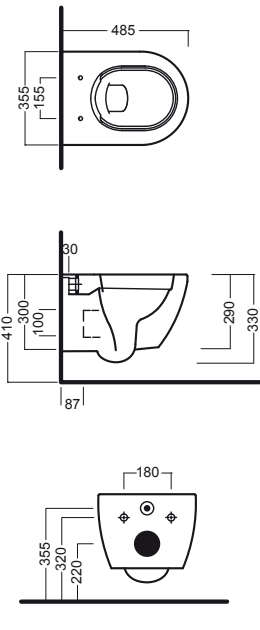
vaso sospeso PURE RIM PURE RIM wall hung wc
