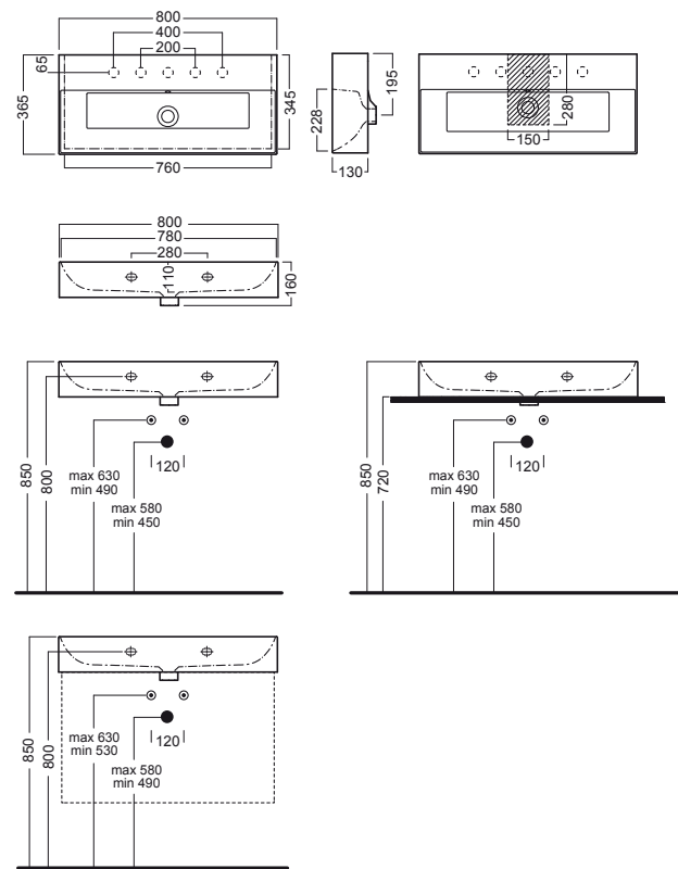
lavabo 80x36,5 washbasin 80x36,5
