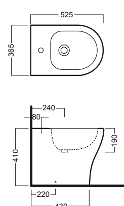
bidet filo muro back to wall bidet
