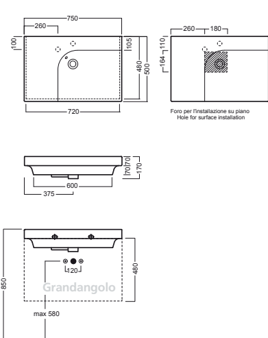
con sifone salvaspazio - with space saver trap_Y1M5
