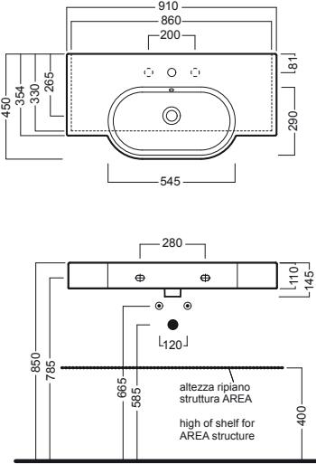
lavabo 90x45 washbasin 90x45
