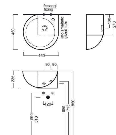
lavabo 46 sinistro washbasin 92 left
