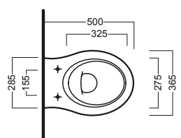
vaso sospeso_50 wall hung wc_50
