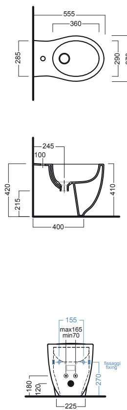
bidet filo muro_OPEN BIDET back to wall bidet_OPEN BIDET
