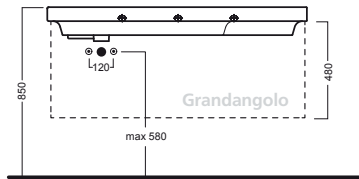
con sifone salvaspazio - with space saver trap_Y1M5
