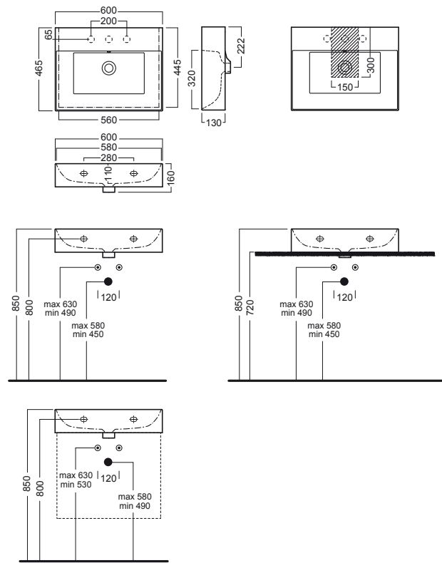
lavabo 60x46,5 washbasin 60x46,5
