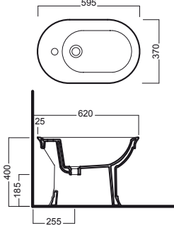
bidet monoforo one hole bidet
