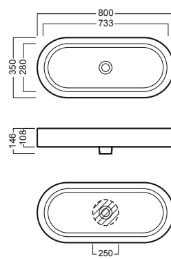
lavabo 80x35 washbasin 80x35
