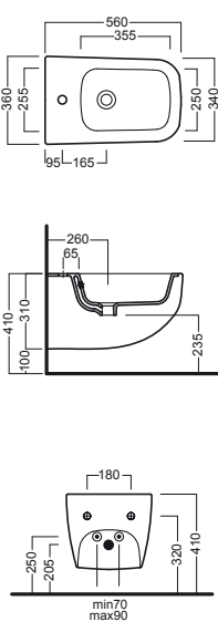
bidet sospeso wall-hung bidet
