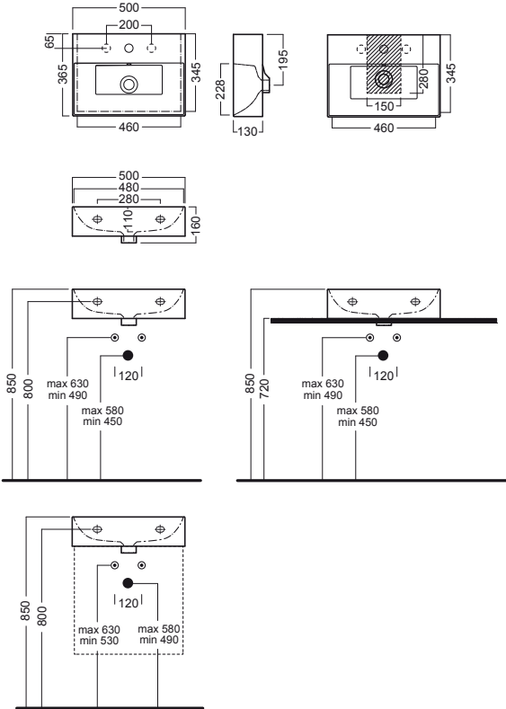
lavabo 50x36,5 washbasin 50x36,5
