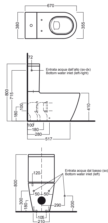
vaso PURE RIM monoblocco con cassetta PURE RIM coupled wc with cistern
