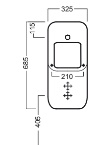
orinatoio sospeso con coperchio wall hung urinal with cover
