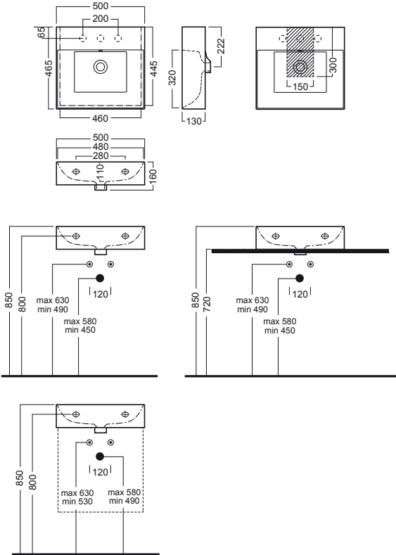
lavabo 50x46,5 washbasin 50x46,5
