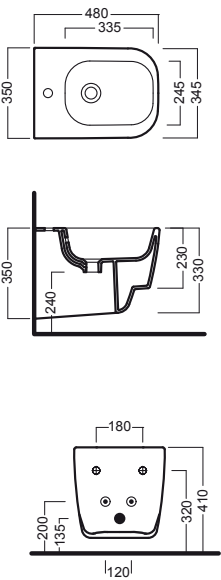
bidet sospeso wall hung bidet
