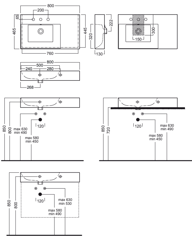
lavabo 80x46,5 destro washbasin 80x46,5 right
