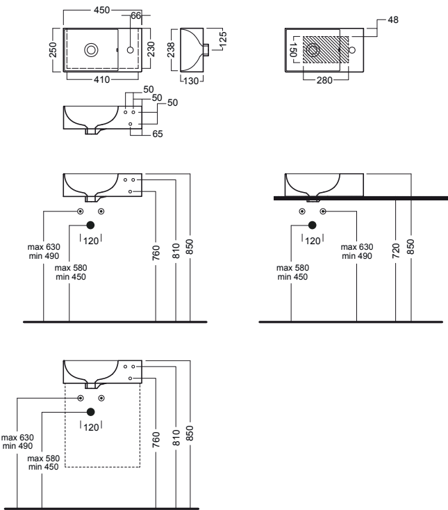
lavamani 45x25 handrinse basins 45x25
