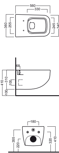
vaso sospeso PURE RIM PURE RIM wall-hung wc
