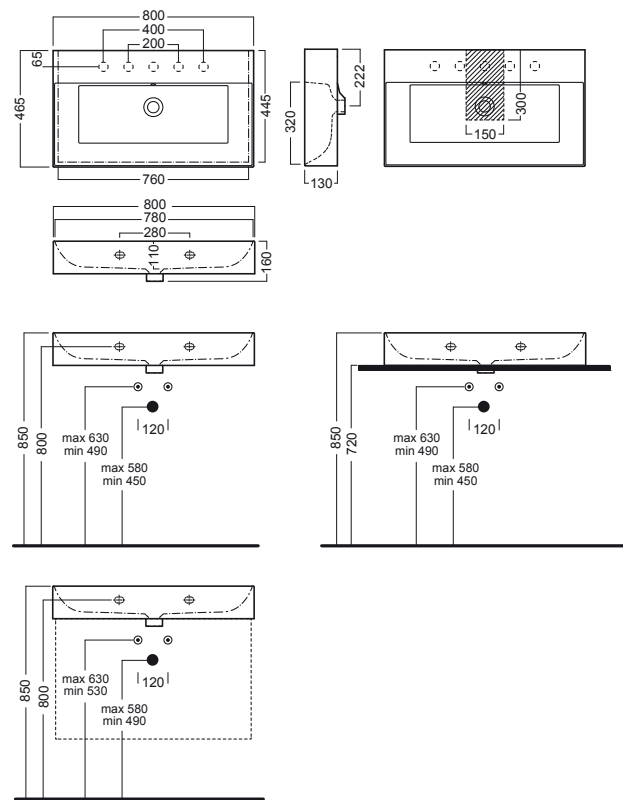
lavabo 80x46,5 washbasin 80x46,5
