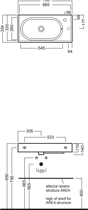
lavabo 70x35 washbasin 70x35
