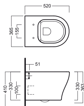
vaso sospeso PURE RIM PURE RIM wall hung wc
