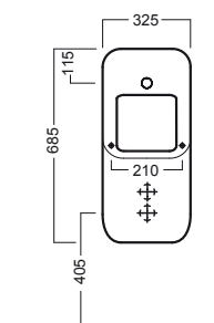
orinatoio sospeso wall hung urinal
