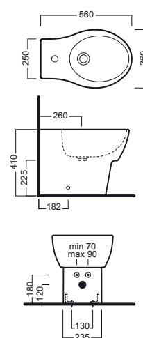
bidet filo muro back to wall bidet
