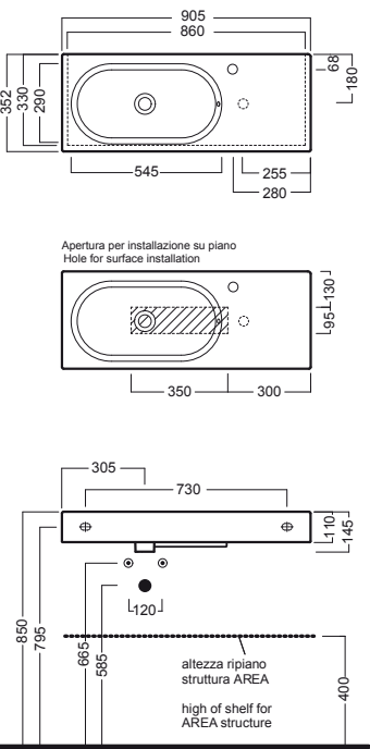
lavabo 90x35 washbasin 90x35
