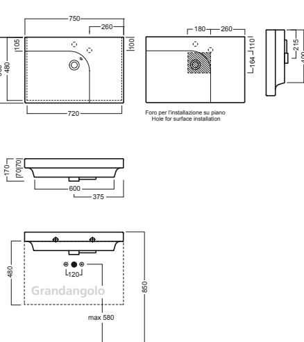
con sifone salvaspazio - with space saver trap_Y1M5
