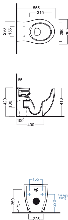
vaso filo muro PURE RIM PURE RIM back to wall wc
