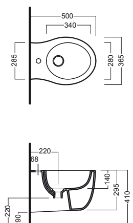
bidet sospeso_50 wall hung bidet_50
